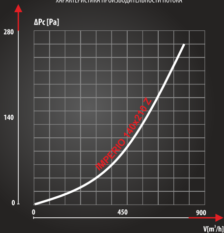
CHARAKTERYSTYKA PRZEPŁYWOWA CHARACTERISTICS OF THE FLOW EFFICIENCY ХАРАКТЕРИСТИКА ПРОИЗВОДИТЕЛЬНОСТИ ПОТОКА
