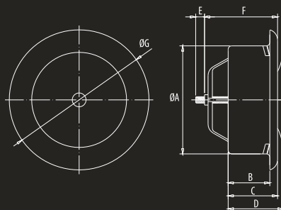
WYMIARY / DIMENSIONS / РАЗМЕРЫ
