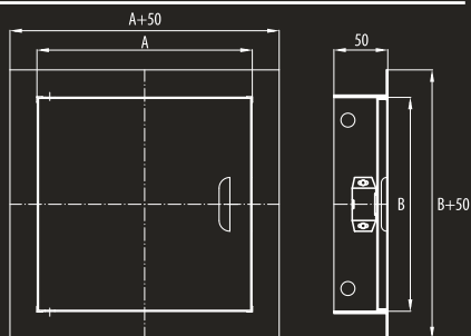
WYMIARY / DIMENSIONS / РАЗМЕРЫ
