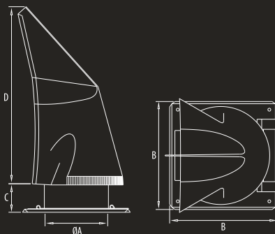
WYMIARY / DIMENSIONS / РАЗМЕРЫ
