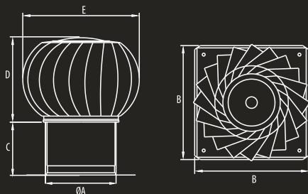
WYMIARY / DIMENSIONS / РАЗМЕРЫ
