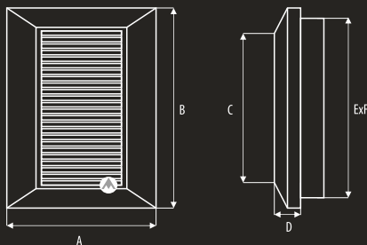
WYMIARY / DIMENSIONS / РАЗМЕРЫ
