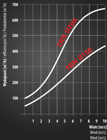
CHARAKTERYSTYKA PRZEPLYWOWA CHARACTERISTICS OF THE FLOW EFFICIENCY ХАРАКТЕРИСТИКА ПРОИЗВОДИТЕЛЬНОСТИ ПОТОКА
