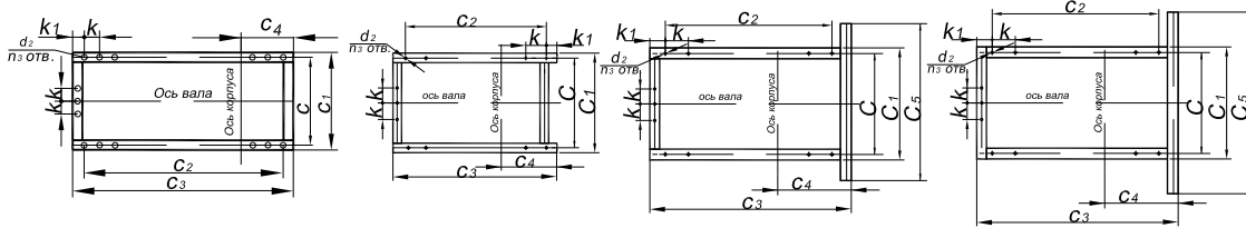
Схемы положений корпуса вентилятора
