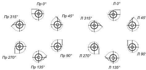
Схемы положений корпуса вентилятора
