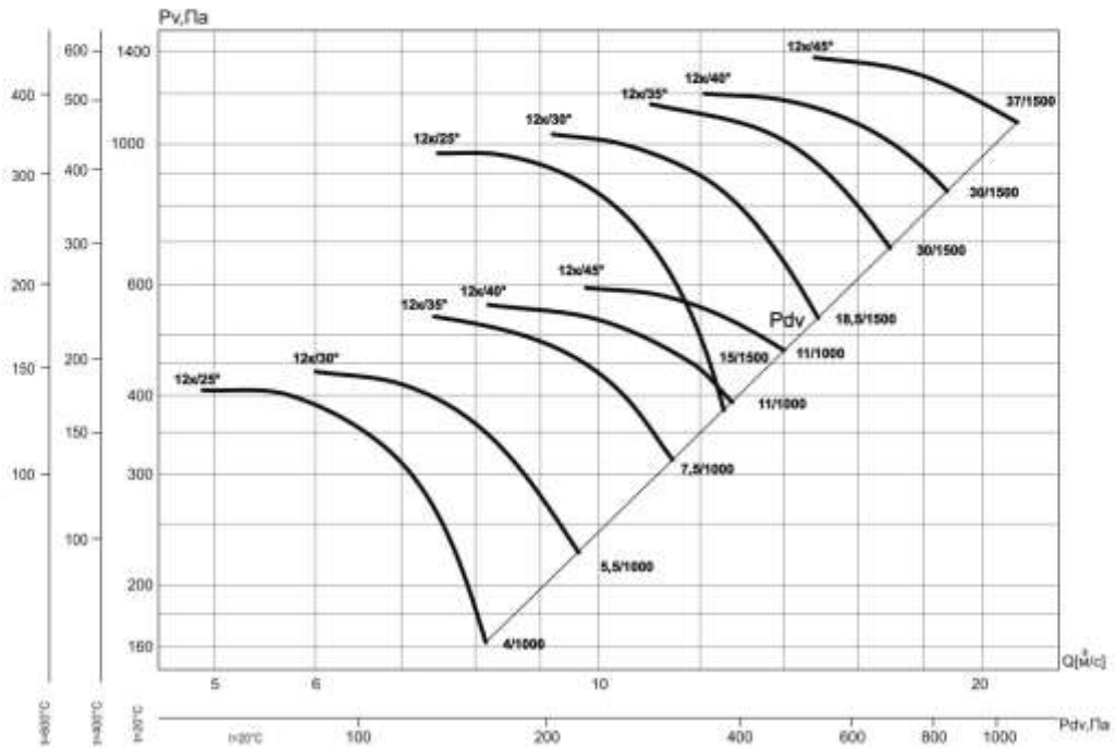
ВО-13-284-12к/(25°, 30°, 35°, 40°, 45°)-10ДУ
