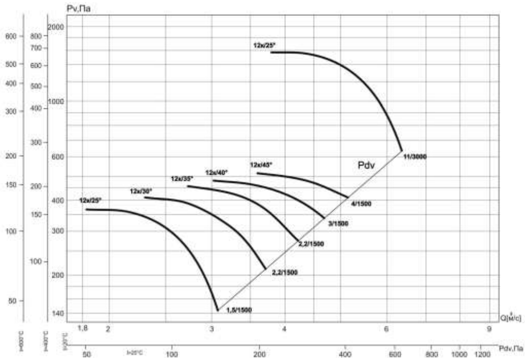
ВО-13-284-12к/(25°, 30°, 35°, 40°, 45°)-6,3ДУ
