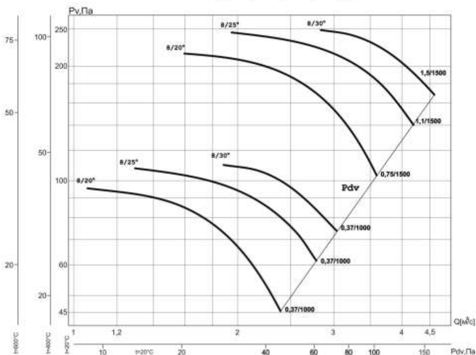
ВО-13-284-8/(20°, 25°, 30°)-6,3ДУ
