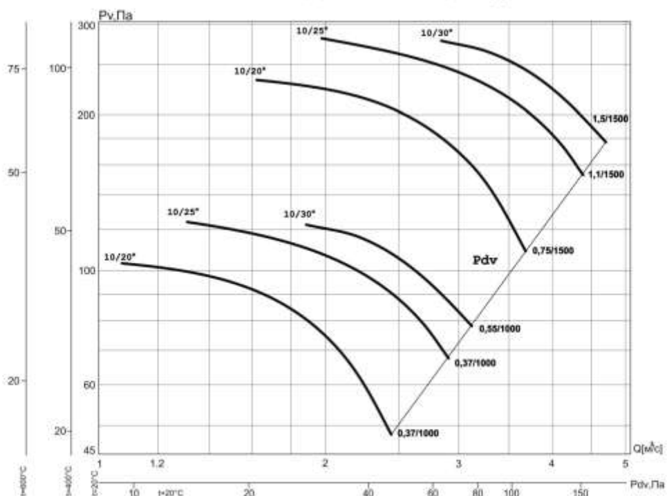
ВО-13-284-10/(20°, 25°, 30°)-6,3ДУ
