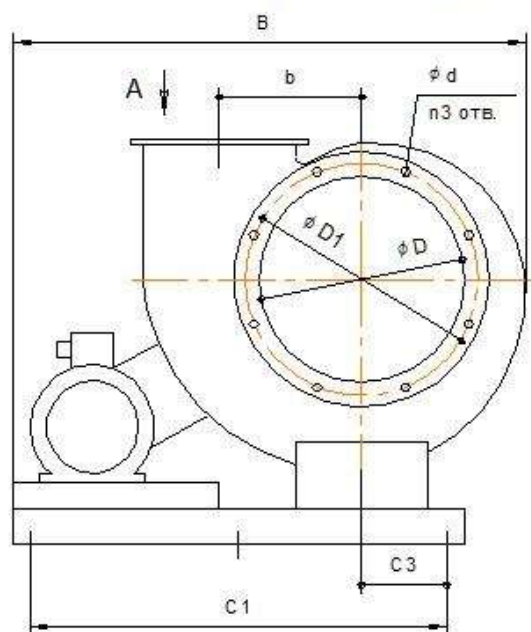
Схема расположения отверстий под фундаментные болты
