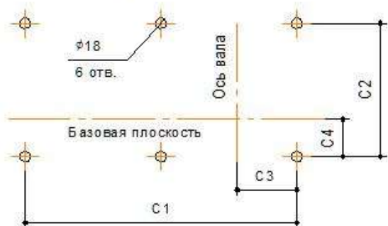
Положения корпуса вентилятора (со стороны входа)
