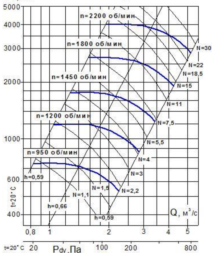
VRP 122-45-6,3 (исп. 1 и 5)
