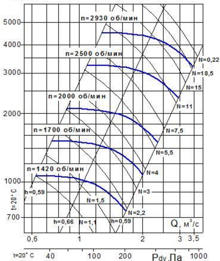
VRP 122-45-5 (исп. 1 и 5)
