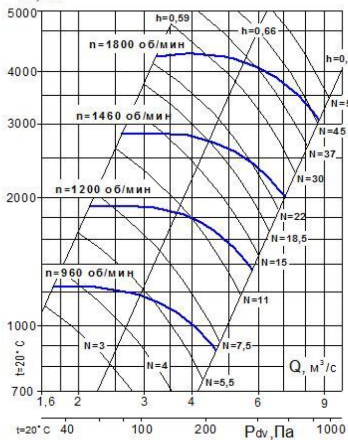
VRP 122-45-8 (исп. 1 и 5)
