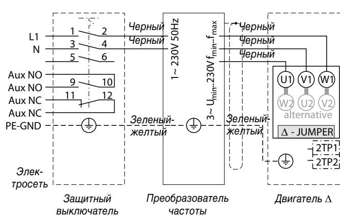
Схема подключения 4
