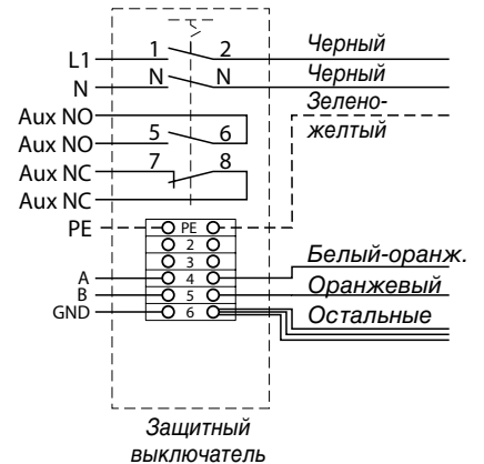
Схема подключения 6
