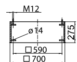
ZKK 20-0071 Прокладка
