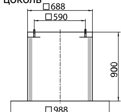
ZBS 09-0071-# Наклонный крышный цоколь
