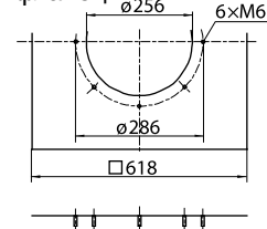
Присоединительный фланец
